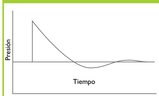
FIGURA 14. Curva de Friedlander
